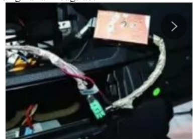
12. Unsere Video-Bildschirm-Umschaltbox wird an das Original-Fahrzeugbildschirmkabel angeschlossen, und das rote Stromkabel wird an unseren Host-Ausgangsstrom ACCOUT angeschlossen.
